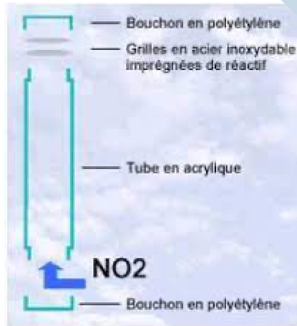
Schéma de fonctionnement du tube absorbant Gradko
