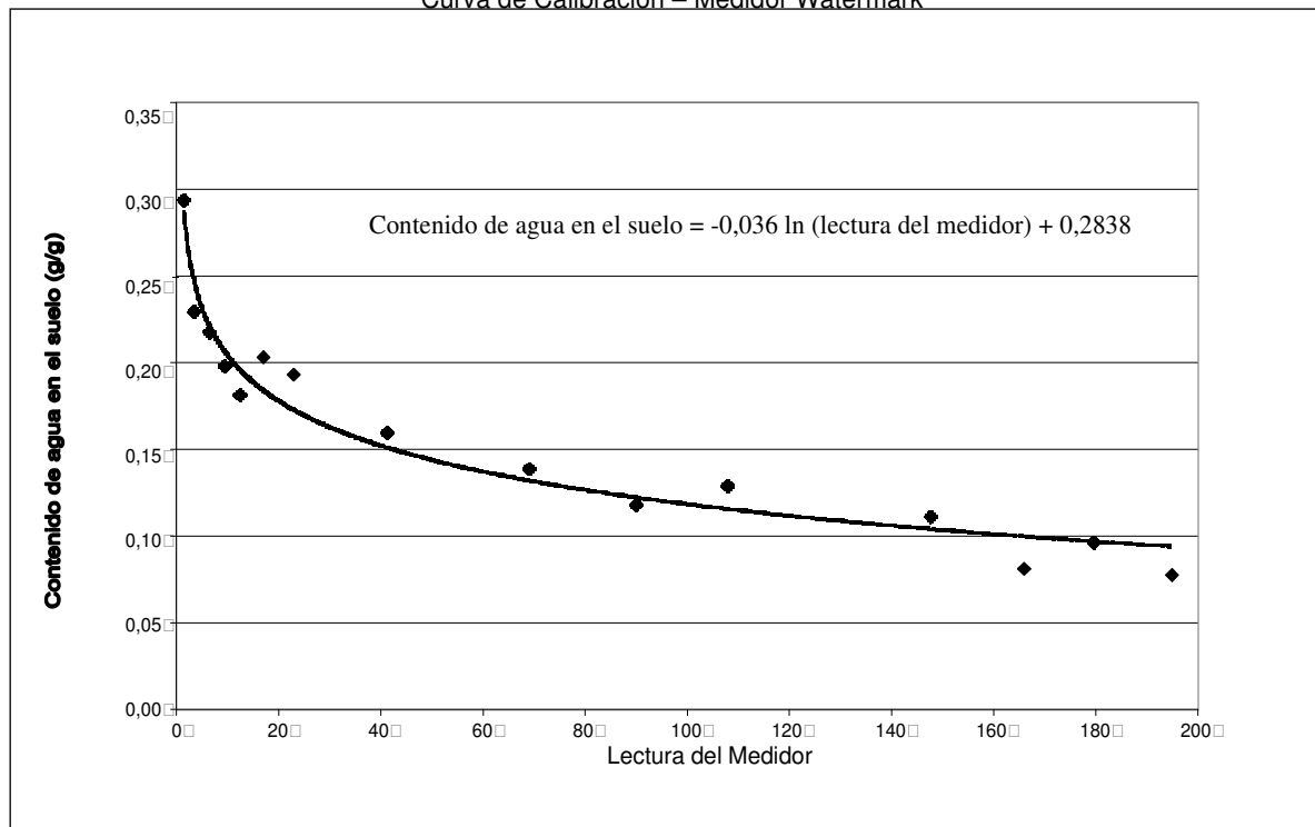
Curva de Calibración – Medidor Watermark
