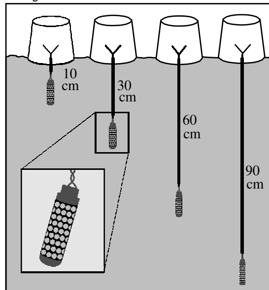
Configuración de los Sensores de Humedad de Suelo Instalados
